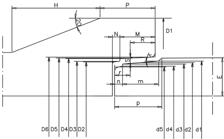
DETALLE ENCHUFE CAMPANA JUNTA ELÁSTOMÉRICA DE LÁGRIMA (mm.)
